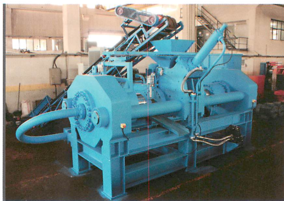
■ bpl Double Ram
